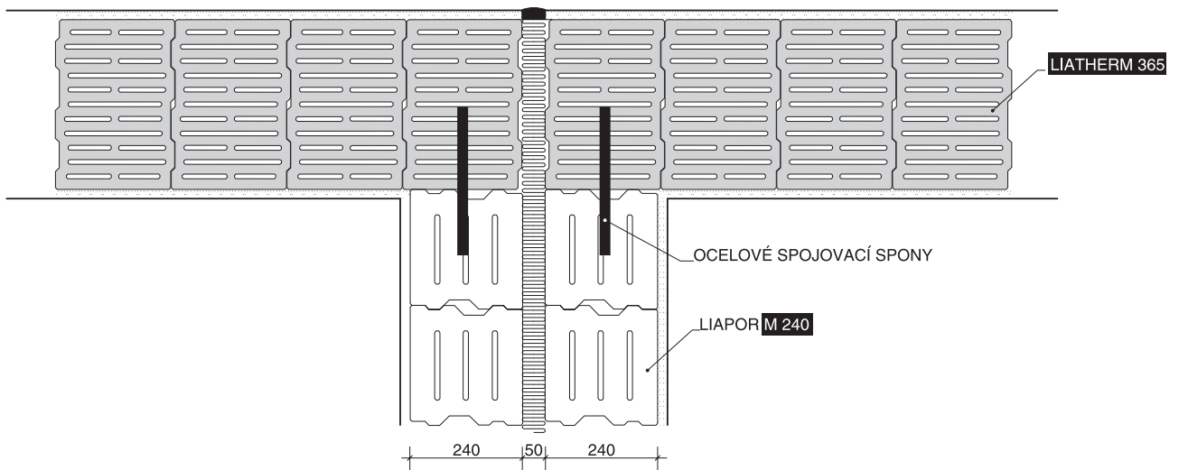
Řešení napojení řadové zástavby v kombinaci Liapor M a Liatherm.
