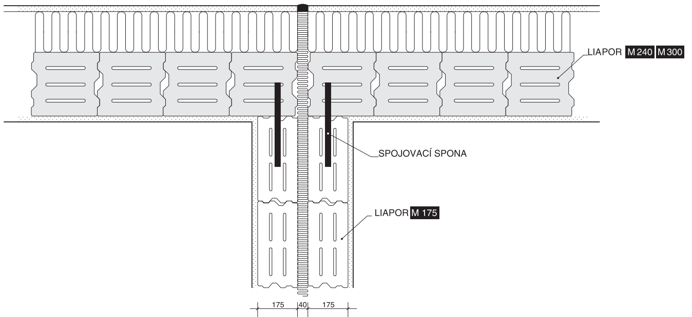
Řešení napojení řadové zástavby v systému Liapor M.
